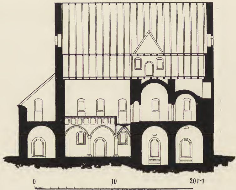
Fig. 280. Querschnitt durch die Kapellen des Chores.
